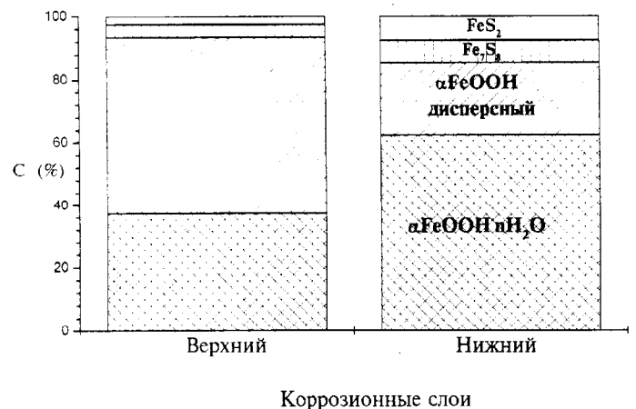
Рис. 5. Процентное содержание фаз в коррозионных слоях осетинского образца, полученное в результате комплексного исследования
