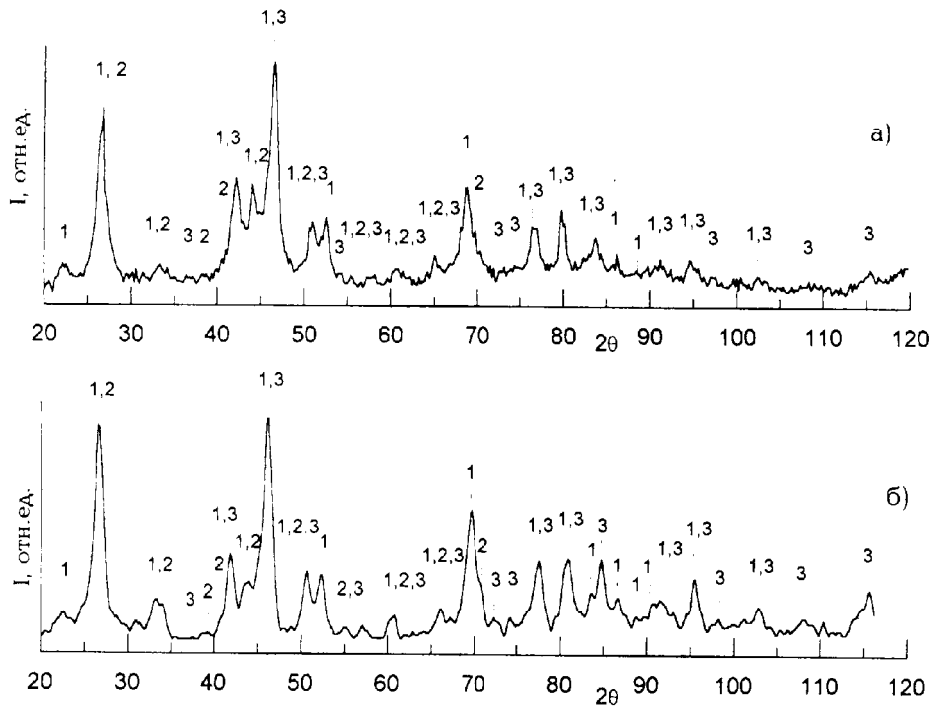
Рис. 1. Дифрактограммы верхней (а) и нижней (б) поверхностей осегиного образца: \alpha -FeOOH (1), \text{CaCO}_3 (2) и \text{FeS}_2 (3)
