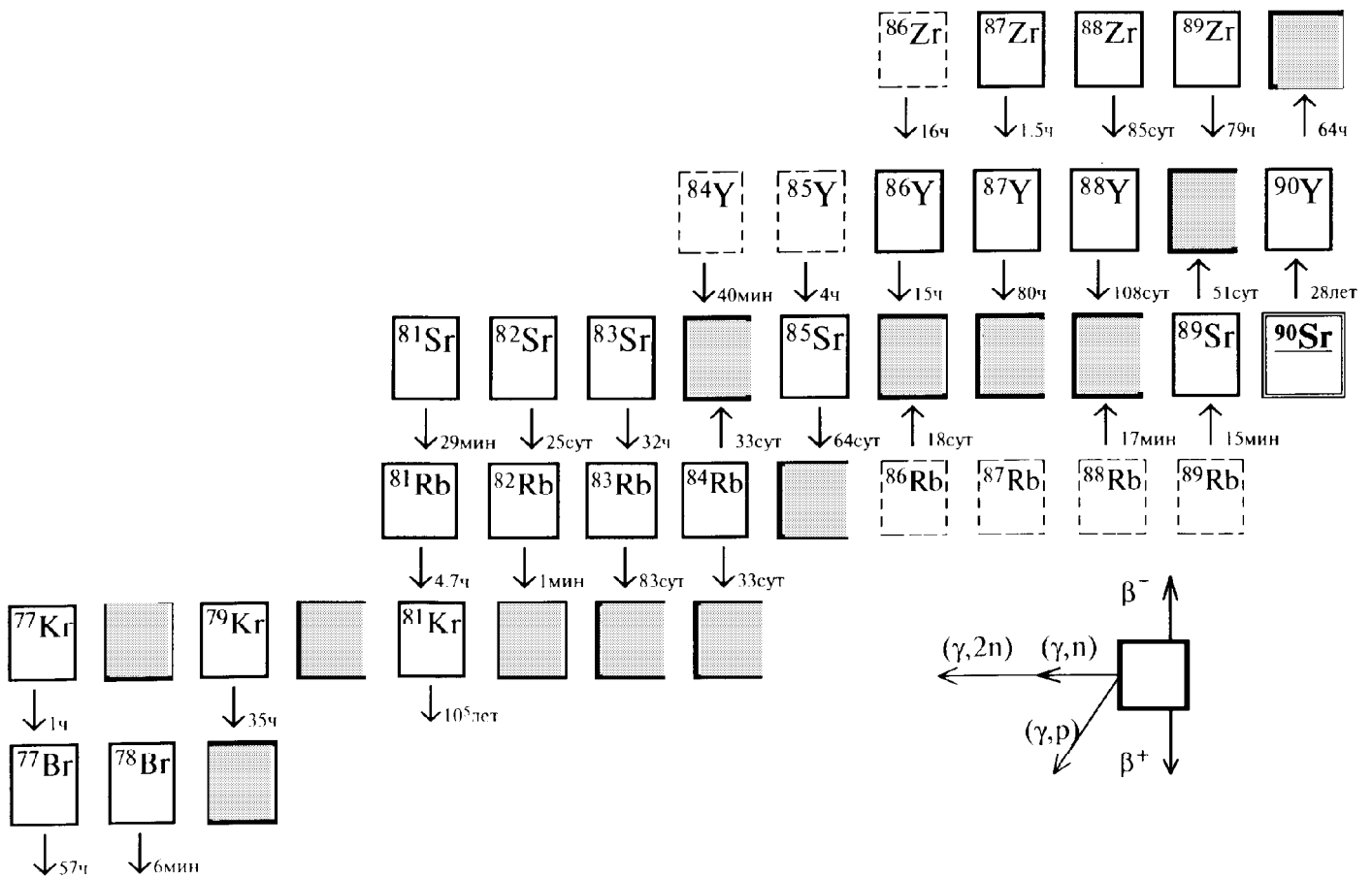
Рис. 1. Трансмутационная цепочка ^{90}\text{Sr} . Запунктированные ячейки — стабильные изотопы, пунктирные — изотопы, образующиеся в результате (\gamma, p) - и (\gamma, 2n) -реакций
