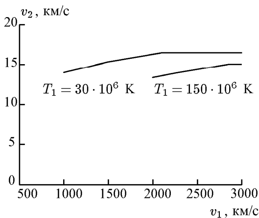
Рис. 1. Зависимость скорости фронта ударной волны v_2 от скорости набегающего потока v_1 при разных температурах T_1
