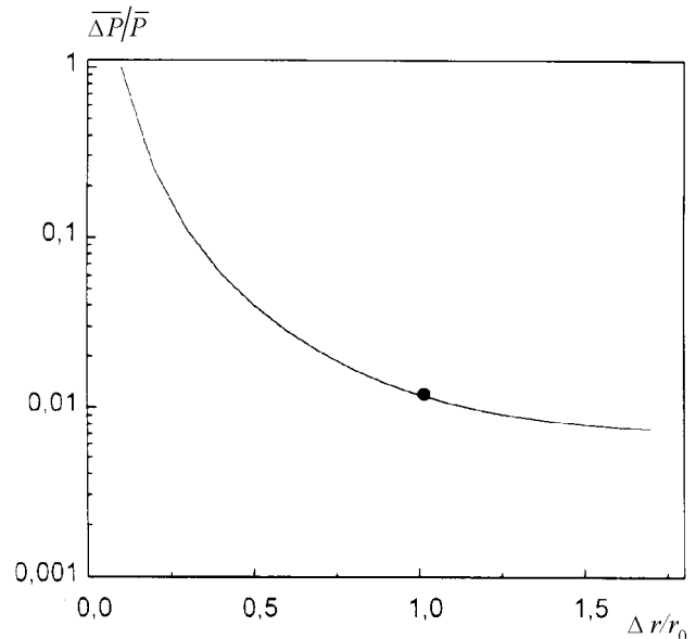
Рис. 3. Зависимость относительной величины низкочастотной нестабильности выходной мощности излучения \Delta \bar{P}/\bar{P} двухволнового лазера от относительного расстояния между осями пучков излучения \Delta r/r_0 при (\Delta^+ \alpha)/(\alpha - 1) = (\Delta^- \alpha)/(\alpha - 1) = 0,005 . Точка на кривой соответствует условиям эксперимента
