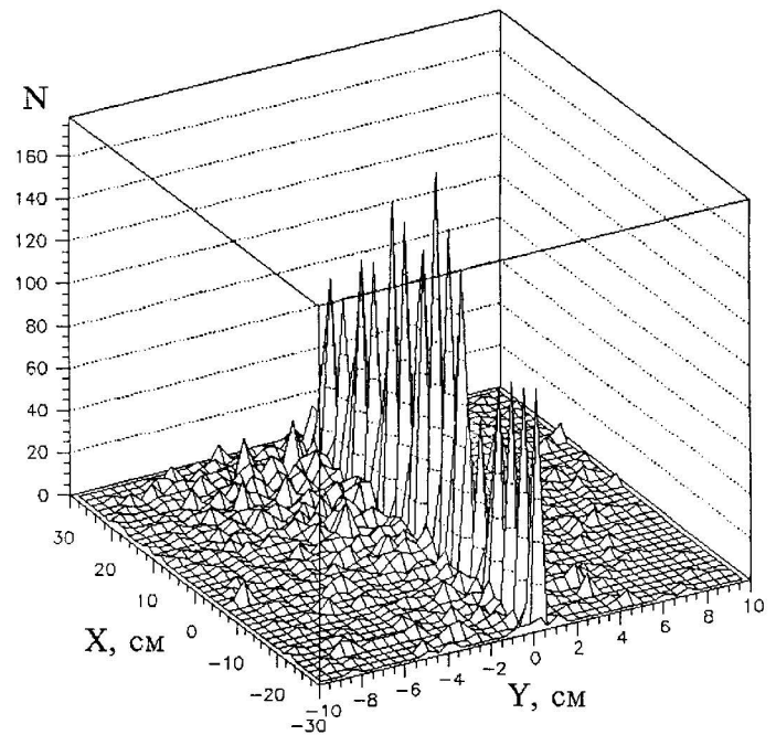
Рис. 2. Пространственное распределение точек пересечения траекторий циркулирующих электронов с плоскостью мишени. Плоскость XU совпадает с плоскостью мишени, ось X — с направлением дрейфа частиц вдоль мишени, ось Y — с направлением вдоль магнитного поля. По оси Z отложено число отсчетов
