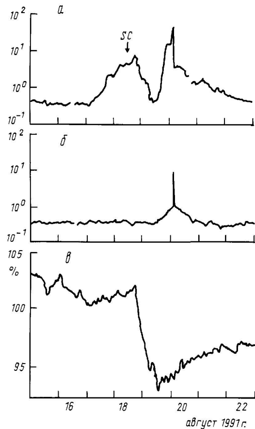
Рис. 1. Потоки протонов ( \text{см}^{-2} \cdot \text{с}^{-1} \cdot \text{ср}^{-1} ) в энергетических интервалах 1–20 МэВ (а) и 5–20 МэВ (б) с антисолнечной стороны; показания нейтронного монитора в Туле (в)
