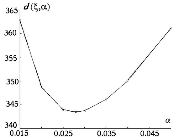
Рис. 2. Статистика d(\xi, \alpha) = \|(I - A(A^*A)^{-1}A^*)\Sigma^{-1/2}\xi\|^2
