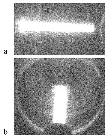
Рис. 1. Общий вид поверхностного СВЧ-разряда на диэлектрическом теле прямоугольной конфигурации при M = 2 , p = 40 Тор, \tau = 50 мкс и f = 100 Гц ( a — вид сбоку, b — вид сверху под углом 45^\circ к вертикали)
