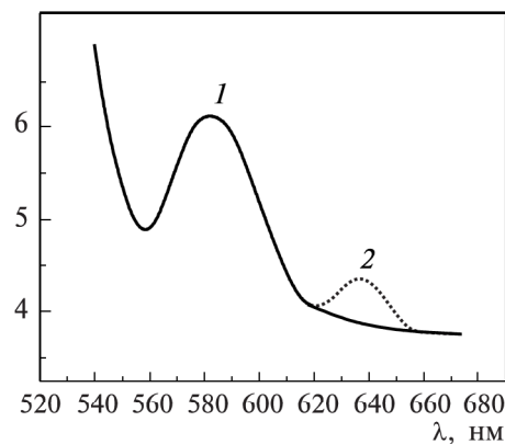
Рис. 1. Характерный вид спектра люминесценции молекул родамина В, адсорбированных на полистироле: 1 — полоса мономеров, 2 — полоса димеров. Слева — спад линии возбуждения
