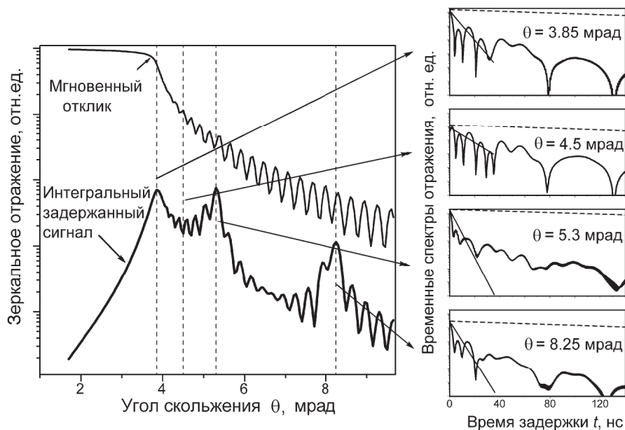
Рис. 1. Рассчитанные кривые РР и ЯРО для структуры [^{56}\text{Fe}(4\text{ нм})/^{57}\text{Fe}(8\text{ нм})]_{10} на кремниевой подложке. Абсолютные интенсивности этих двух кривых зависят от разных параметров: РР — от интегральной падающей интенсивности по всему спектру падающего излучения, ЯРО — от спектральной плотности в резонансной области. Справа показаны временные спектры ЯРО в логарифмическом масштабе для разных углов скольжения. На этих спектрах пунктирная линия представляет естественный распад, а точечные линии показывают ускорение коллективного распада в начальный момент, изменяющееся с углом скольжения. При расчетах предполагалось, что на ядрах ^{57}\text{Fe} имеется сверхтонкое магнитное поле 32 Т с распределением 3 Т, а намагниченность ориентирована в плоскости пленки (планарная анизотропия)
