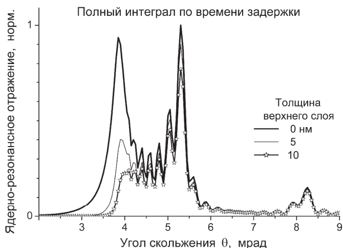
Рис. 5. Влияние наличия поверхностного нерезонансного слоя различной толщины на кривые отражения ЯРО от идеальной структуры. Остальные расчетные параметры те же, что и для других графиков
