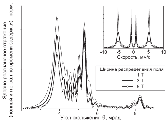
Рис. 3. Рассчитанное изменение кривых ЯРО в зависимости от уширения линий магнитного секстета в мёссбауэровском спектре (приведен в вставке). Нормировка на максимум кривой, рассчитанной для поля с шириной распределения 3 Т
